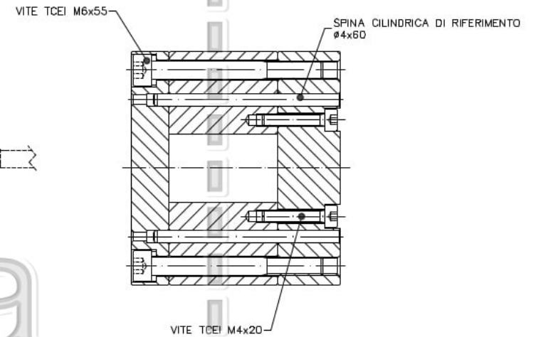
SEZ. B-B
