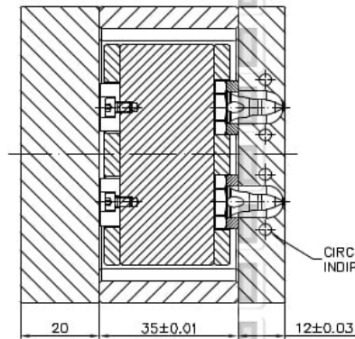
SEZ. C-C
